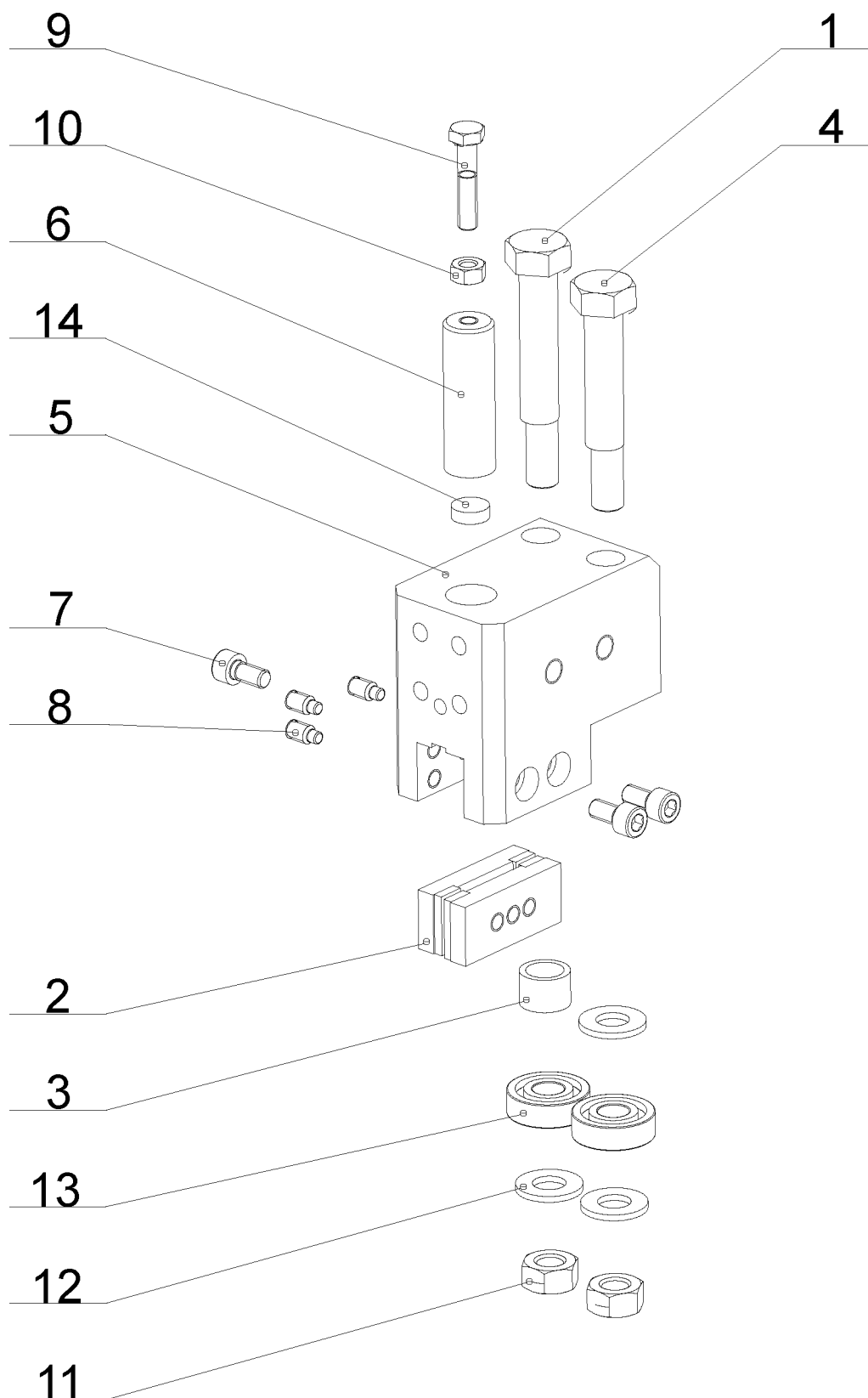
24.12. Pravá vodící kostka / Rechter Führungsklotz / Right guiding cube - individual 410.260 GH
