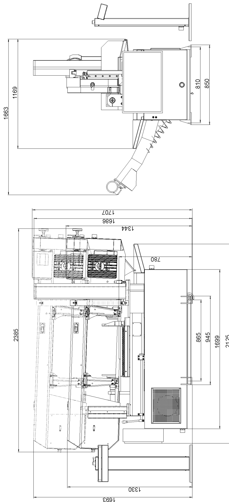
Rozměrové schéma 1 / Aufstellzeichnung 1 / Installation diagram 1 – individual 510.330 GH
